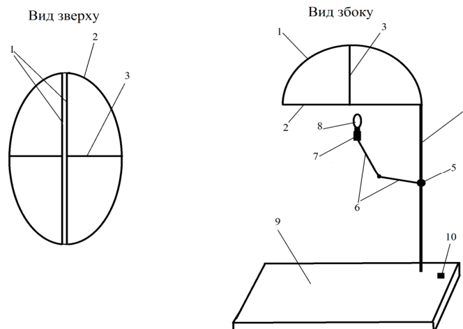
Рис. 4. Пристрій для вивчення вологих препаратів конвексітальної поверхні твердої оболони головного мозку: 1 - пара повздовжніх дугоподібних дротяних стрижнів; 2 - дротяний каркас овальної форми; 3 - пара поперечних дугоподібних дротяних стрижнів; 4 - полий металевий штатив; 5 - гвинт для закріплення гнучкого металевого стрижня; 6 - гнучкий металевий стрижень; 7 - патрон для електричної лампа; 8 - електрична лампа; 9 - дерев'яна основа; 10 - вимикач для світла.
